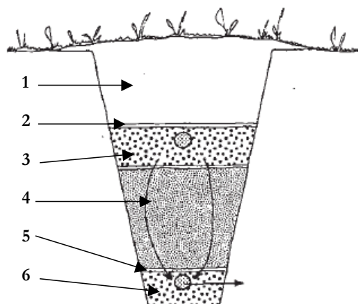
Markbädd (sektion).
